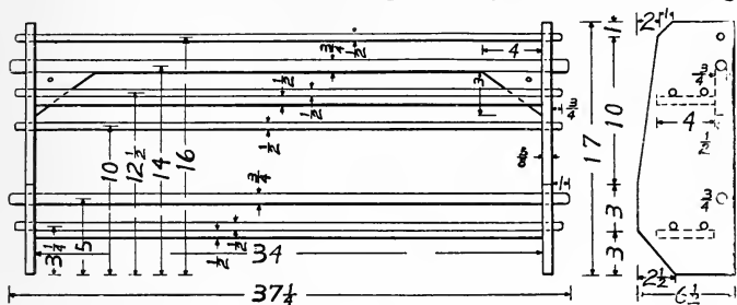
Fig. 238—Plate Rack
